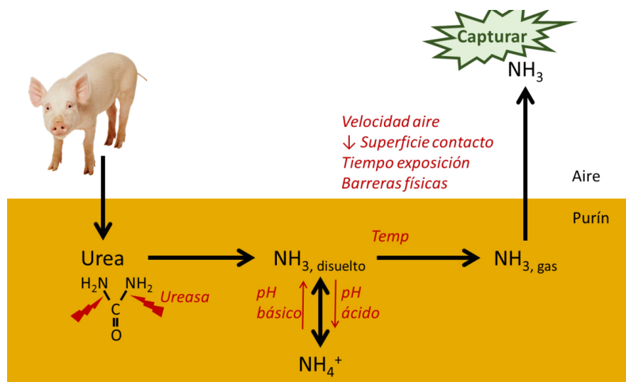
Figura 32. Lugar de acción de los lavadores de aire en la cadena de reacciones de emisión de \text{NH}_3 .
